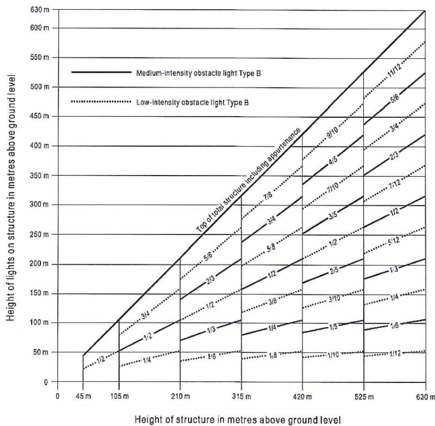
Figura A-2: Sistema de iluminação de obstáculos de média intensidade com luzes vermelhas intermitentes, Tipo B
