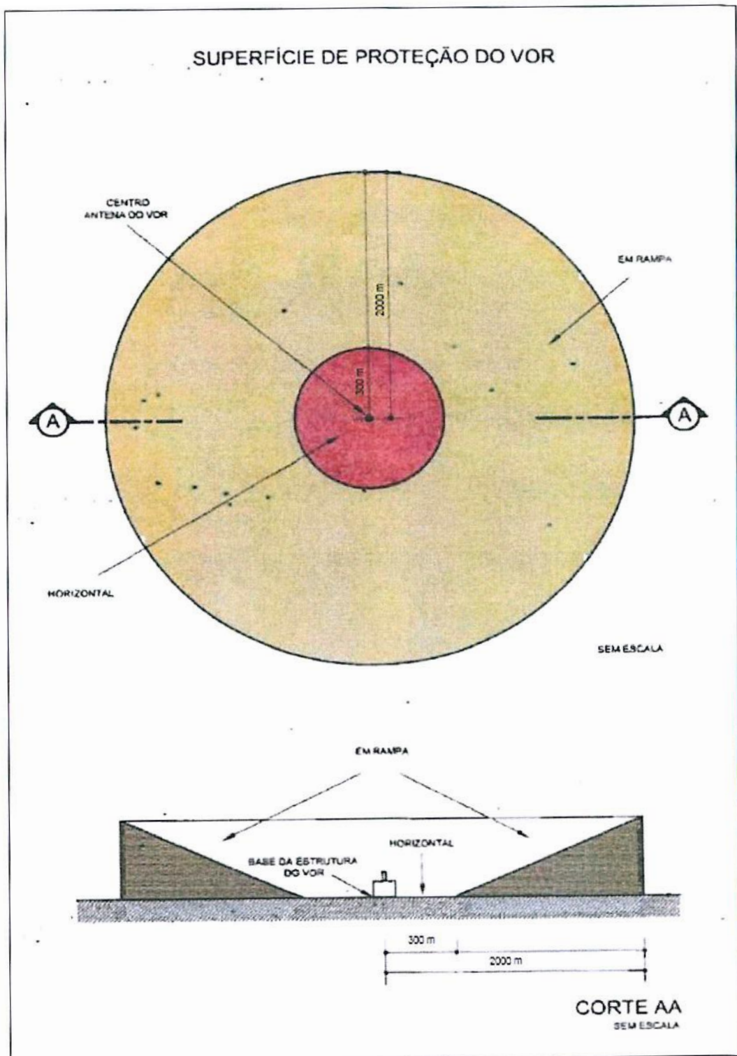
Figura C-3: Superfície de proteção do VOR
