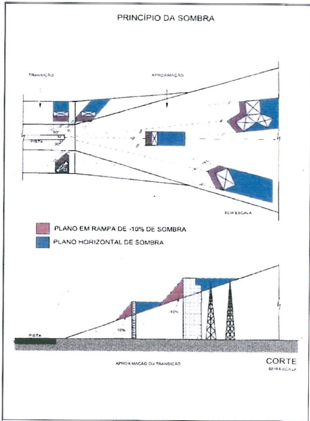
Figura F-1.1: Princípio de sombra
