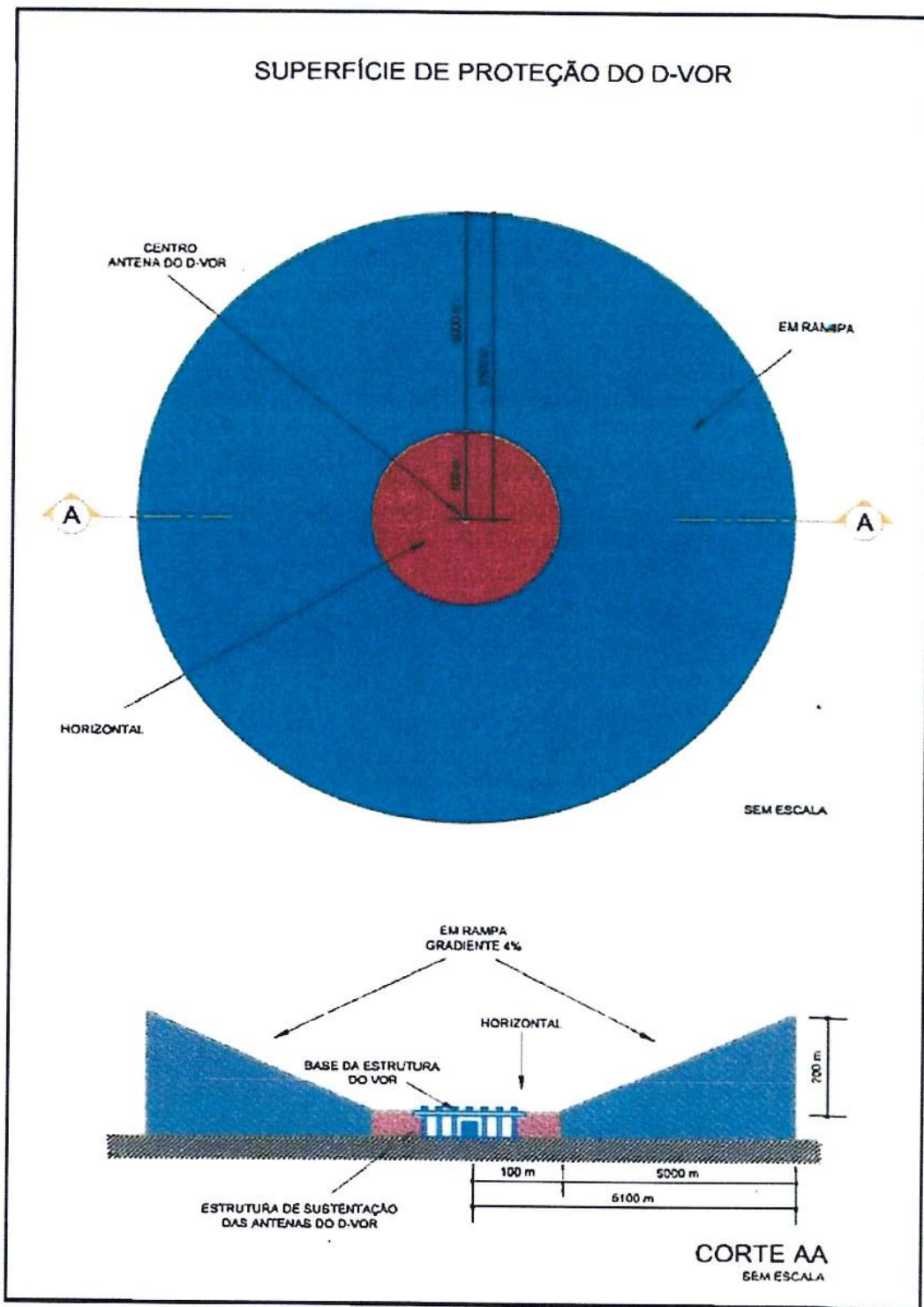
Figura C-4: Superfície de proteção do D-VOR
