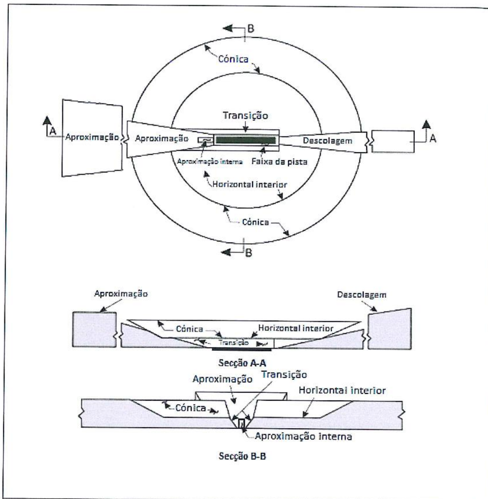
Figura B-1: Superfícies limitadoras de obstáculos
