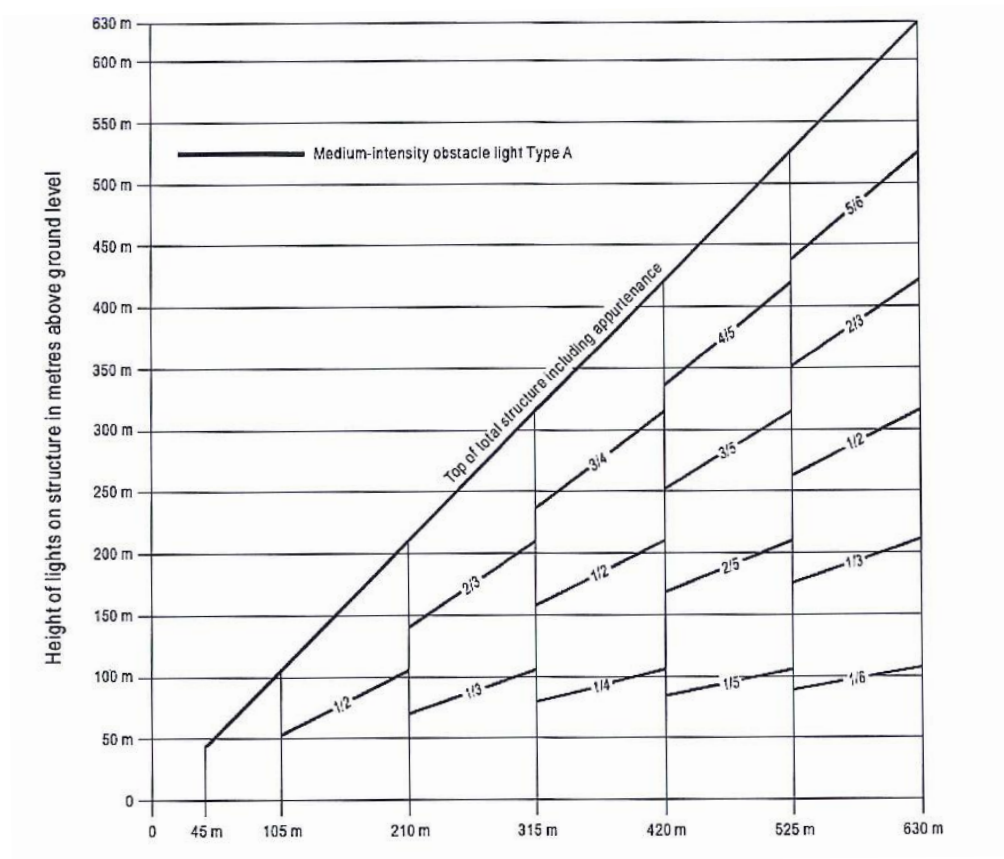
Figura A-1: Sistema de iluminação de obstáculos de média intensidade com luzes brancas intermitentes, Tipo A
